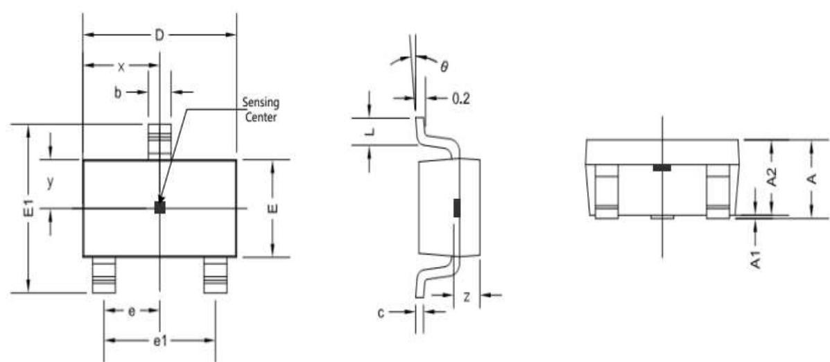
S0T23-3L 封装尺寸
